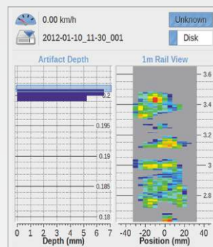
Ausbröckelungen auf dem Gleis und das Abbild im Messprogramm
