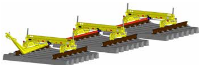
ROLLY 52.16 Ausführung 5 mit Drehschemel, Feststellbremse und Rungen – 8269900040
